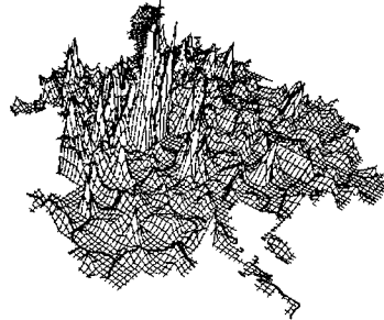
図6 夜間人口分布
