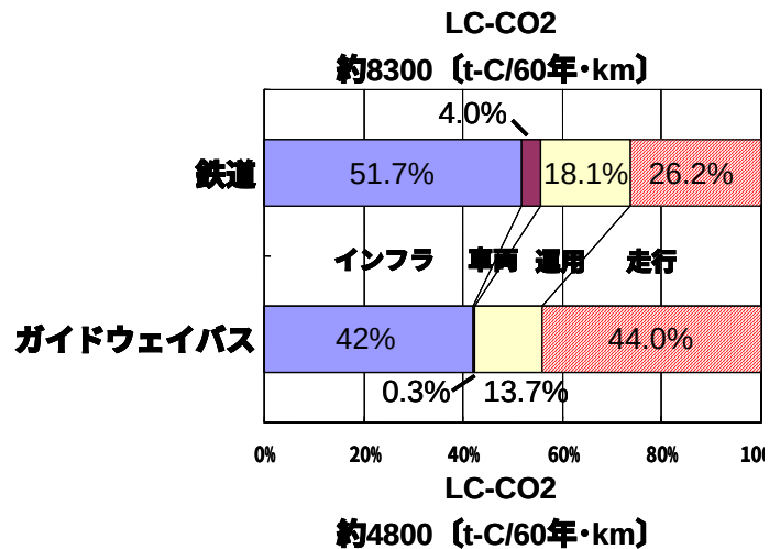
図3 ガイドウェイバス・鉄道の単位距離当たりのLC-CO 2
