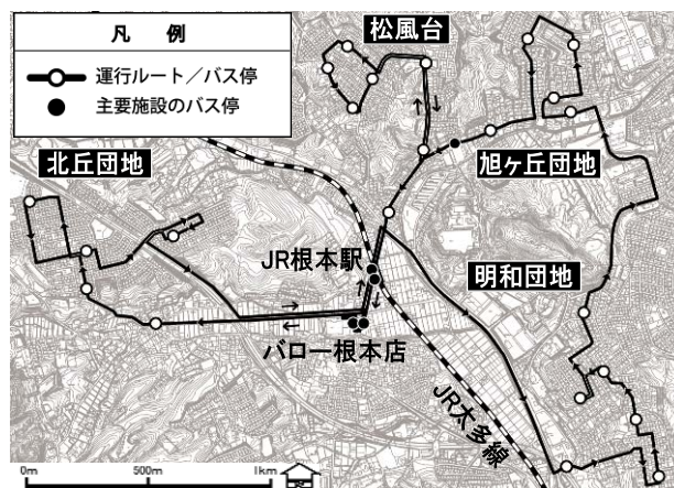
図-2 根本おでかけバスの路線図（運行開始直後）
