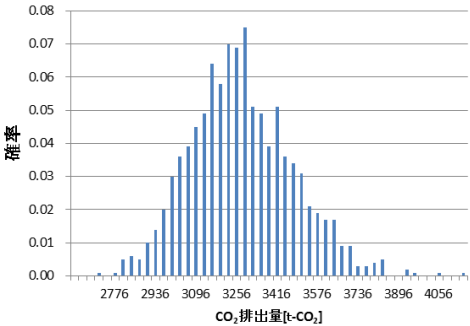
図-3 CO 2 排出量推計結果の確率分布
