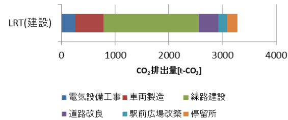
図-2 代表値に基づいたCO 2 排出量推計結果
