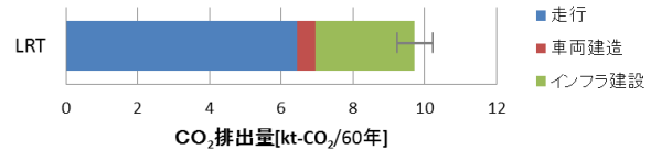
図-5 ライフサイクル CO 2 における建設段階の不確実性
