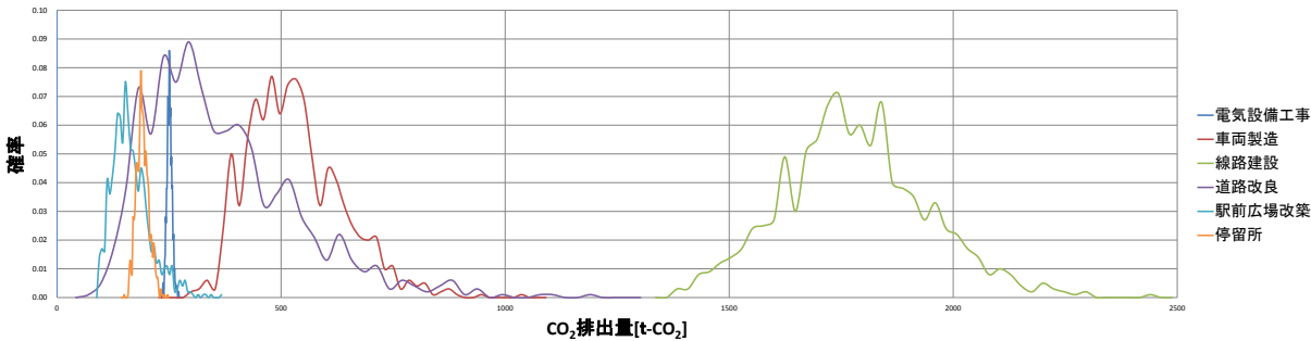
図-4 各項目のモンテカルロシミュレーション結果
